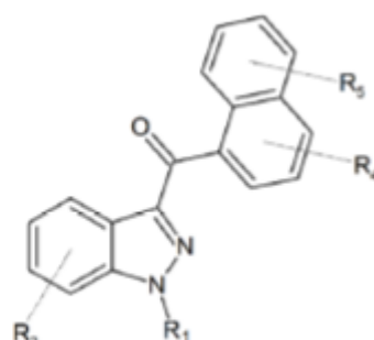
ESTRUTURA B4
