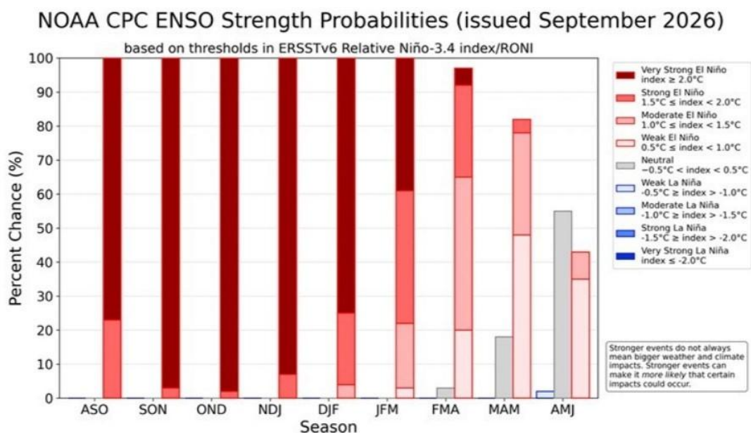
Figura 1 – Probabilidades projetadas de intensidade do El Niño para os trimestres móveis entre agosto de 2026 e junho de 2027.
